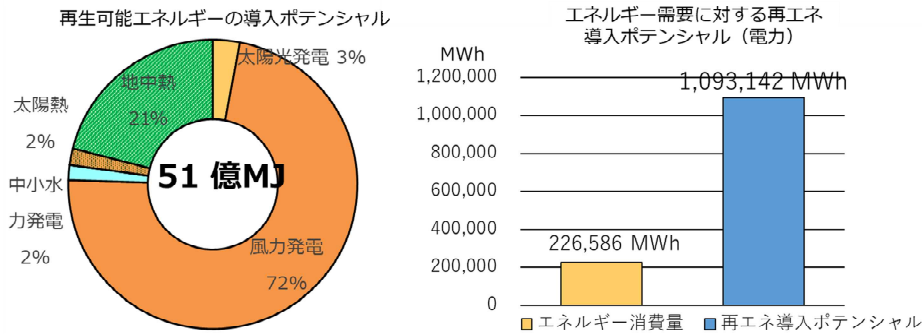
図 11. 北広島町の再生可能エネルギーの導入ポテンシャル
