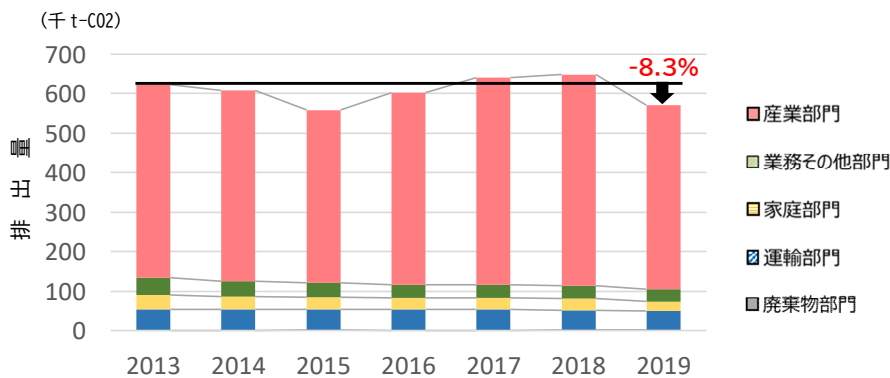
図 15. 部門別二酸化炭素排出量の推移
