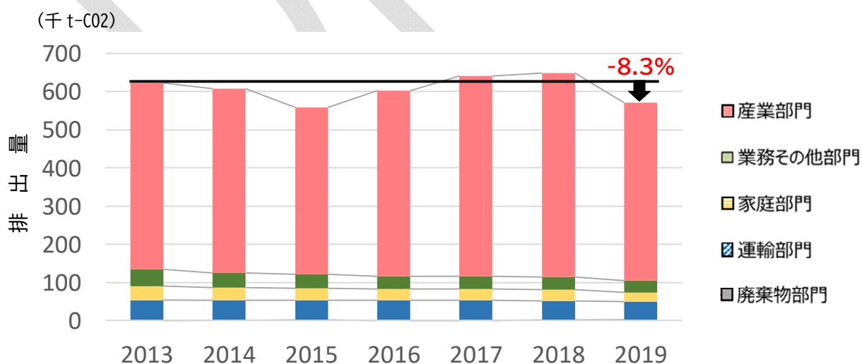
図●. 部門別二酸化炭素排出量の推移
