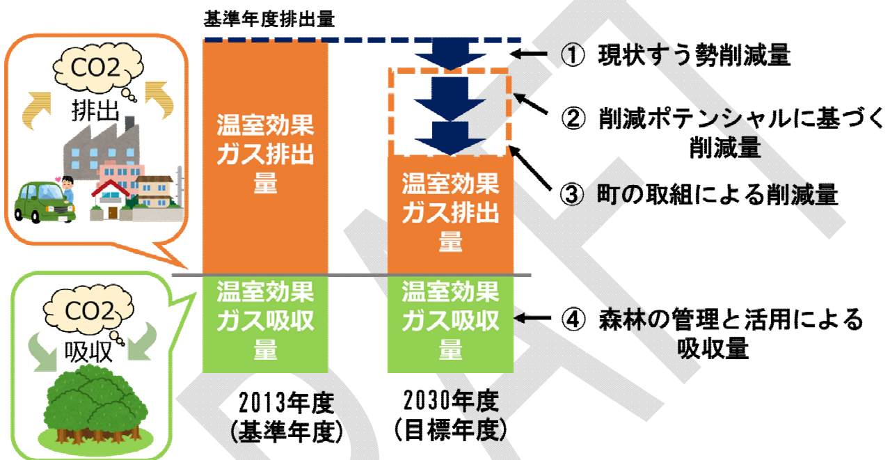
図●. 目標達成に向けた二酸化炭素の排出削減量と吸収量の考え方
