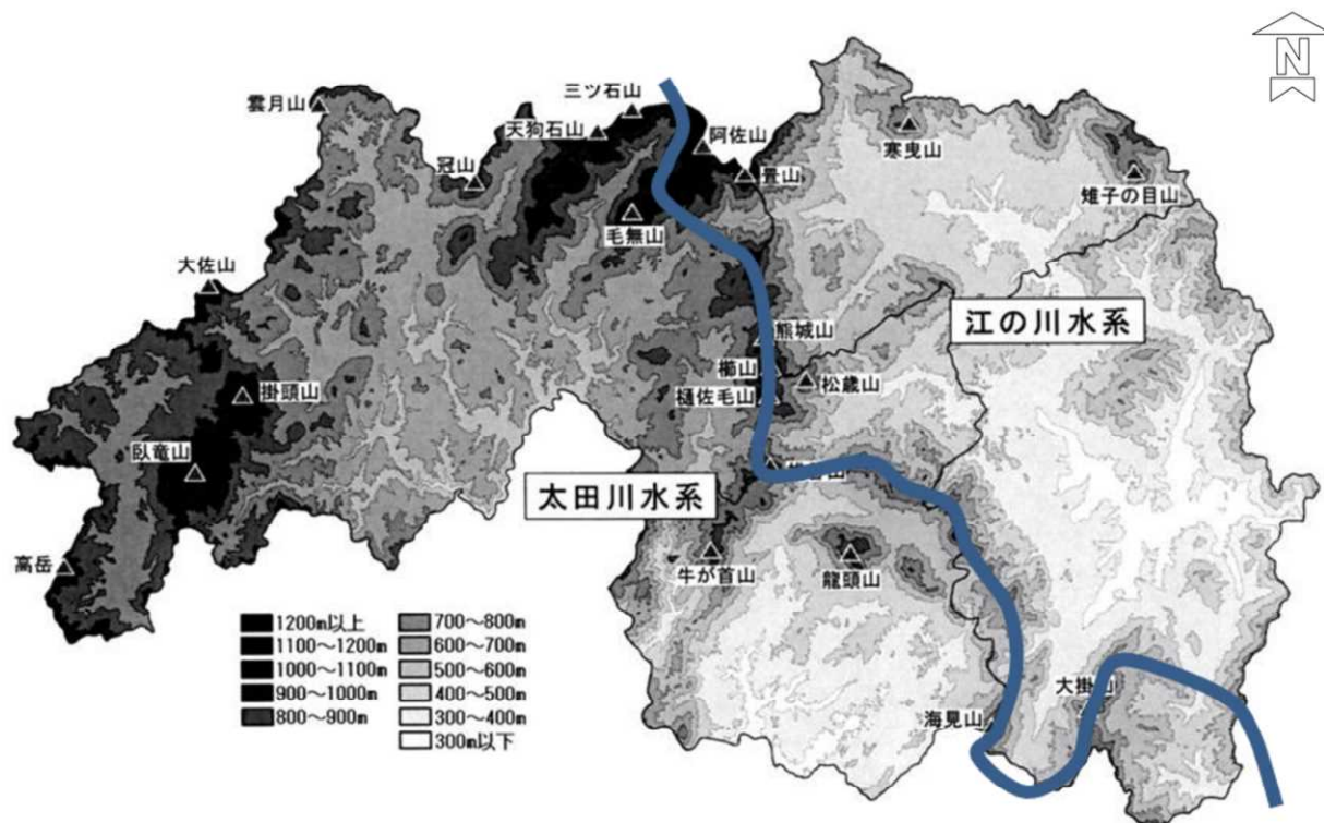
図●. 北広島町の地形と標高
