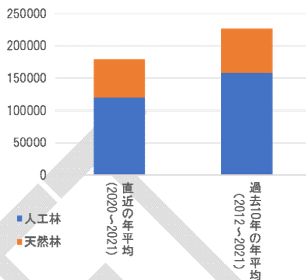
図● 町内森林による二酸化炭素吸収量の比較
