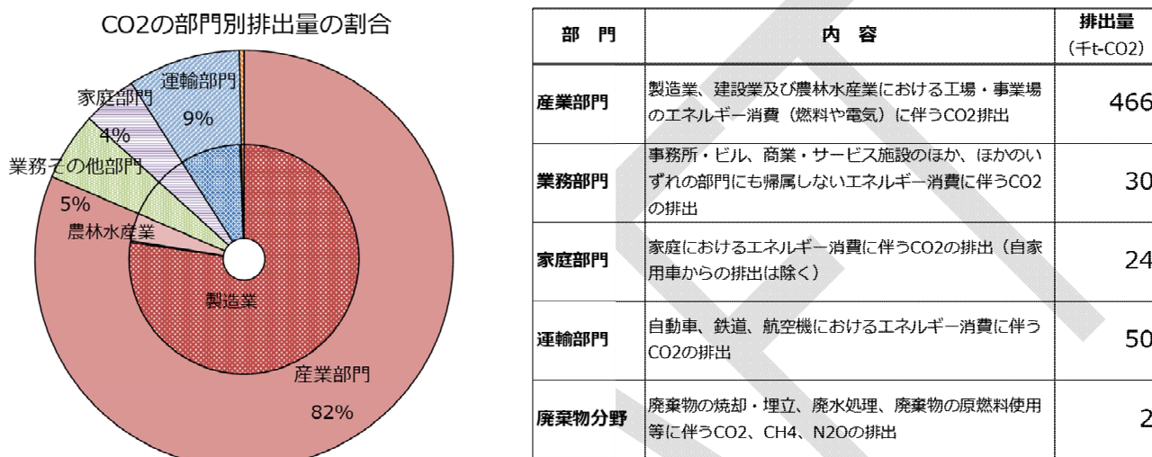
図●. 北広島町の二酸化炭素排出量の部門別内訳（2019年度）
