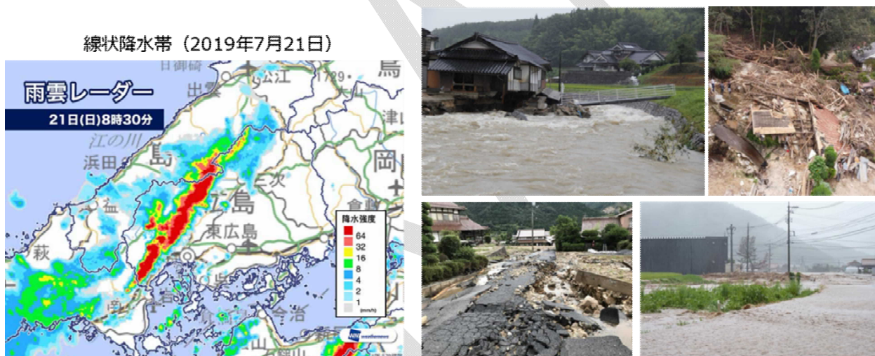
図●．北広島町における地球温暖化の影響
