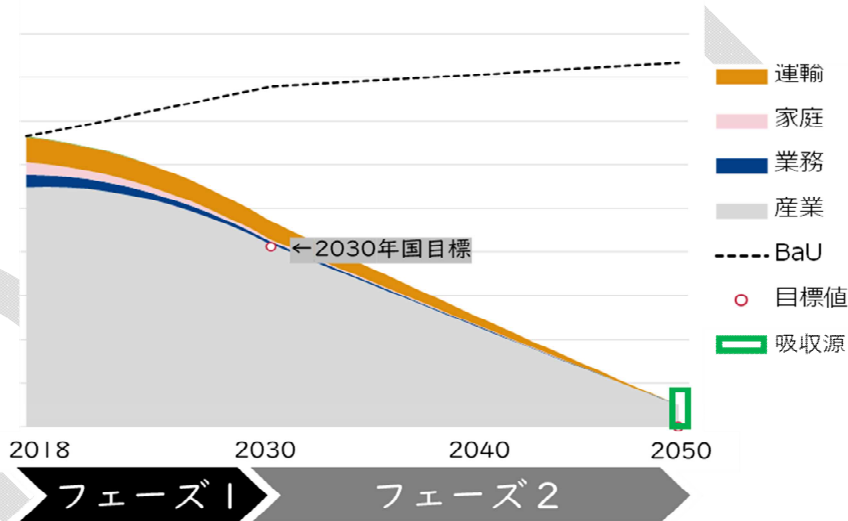
区域全体・CO2排出量推移（部門別）
