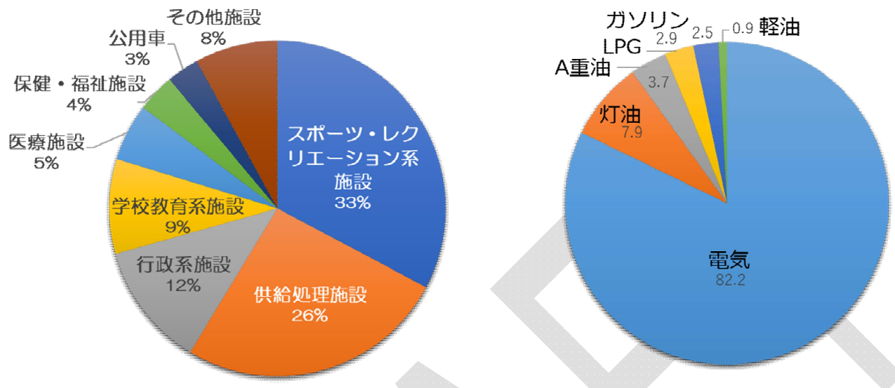
図●. 施設種別（左）とエネルギー種別（右）の温室効果ガス排出量の割合
