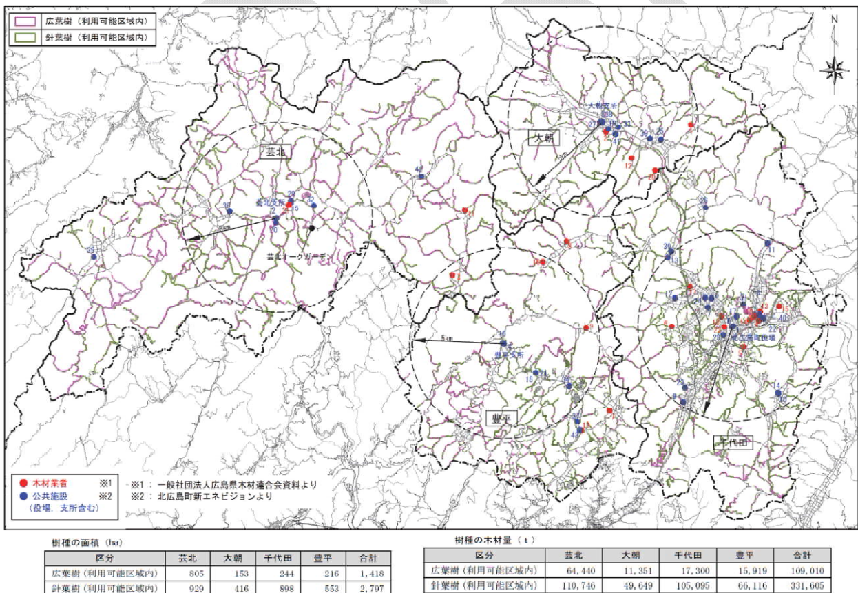
図●. 北広島町樹種別分布図・木材利用可能量
