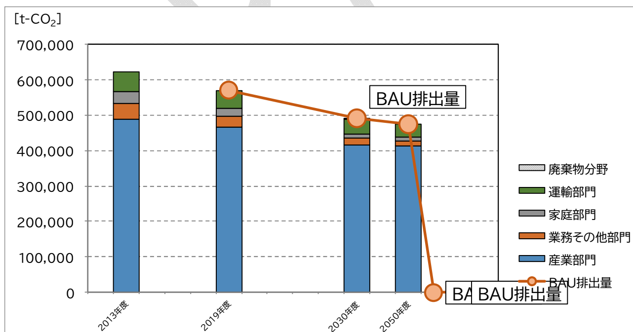
図●. 現状すう勢 (BAU) 及び電力排出係数の削減量を加味した場合の二酸化炭素排出量の推移
