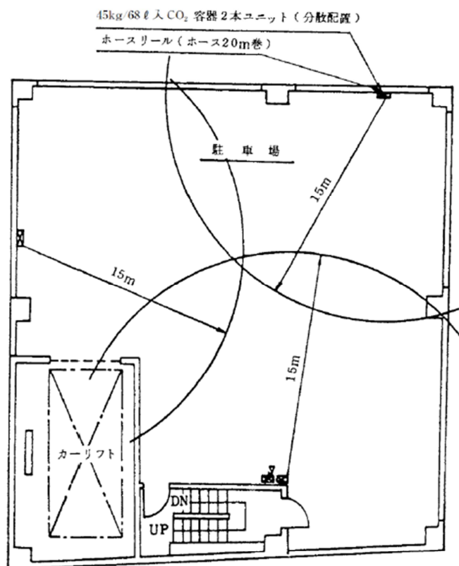
平面図
