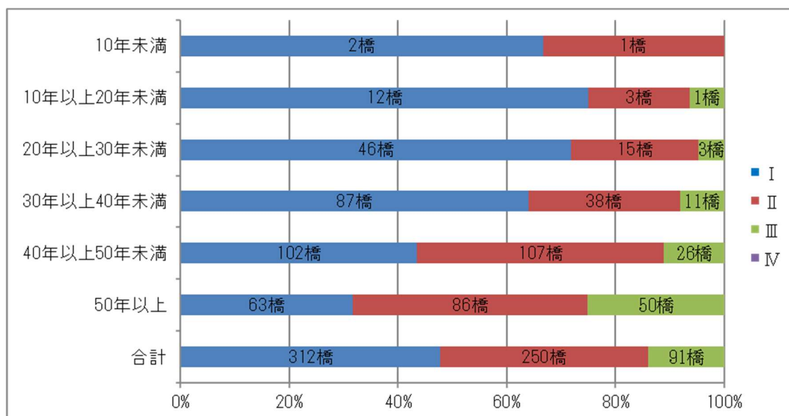
図 1-8 判定区分と建設経過年度
