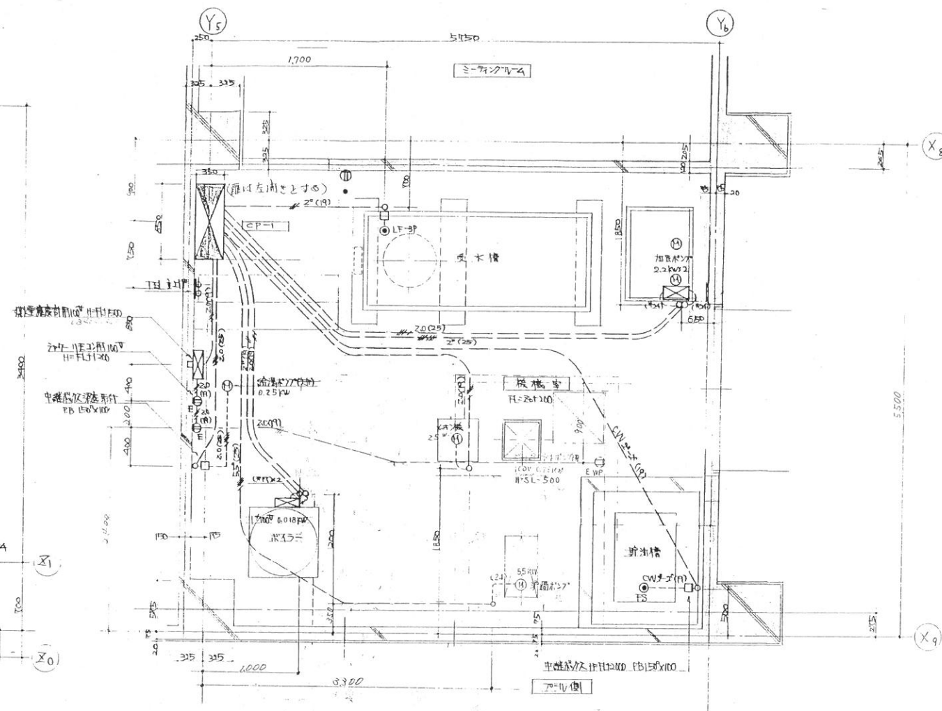
機械室詳圖 図 5-130
