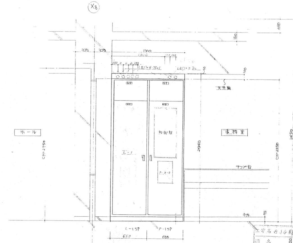
機械室詳圖 図 5-130
