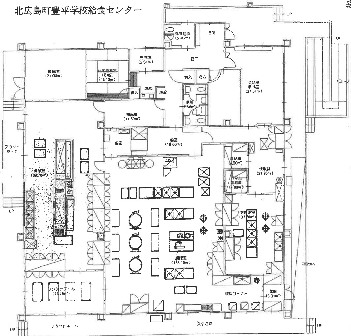
1 階 平 面 図
