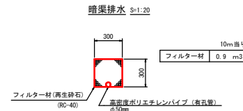
暗渠排水 S=1:20
