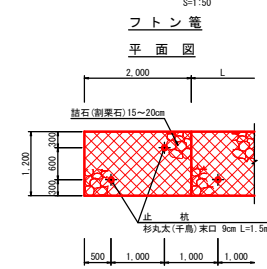
構造図
