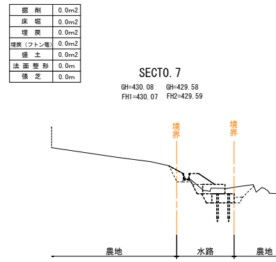
暗渠排水 S=1:20
