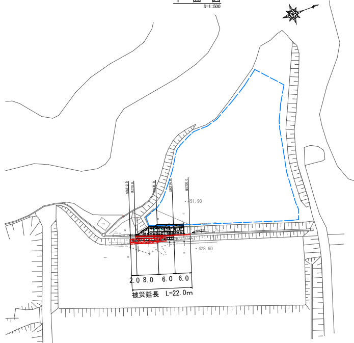
平面図 S=1:500
