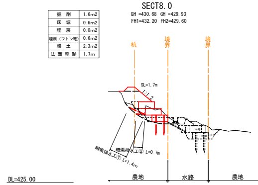
横断面図 S=1:100
