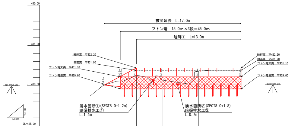
縦断面図
