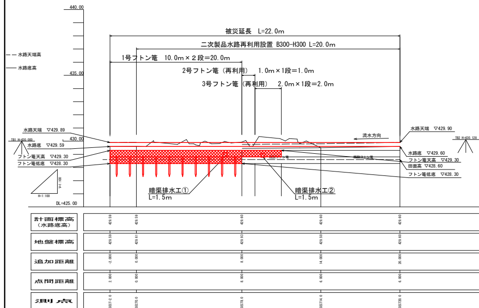
縦断面図
